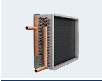
KONDENSORER
